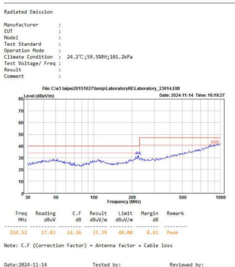
图 6-6 辐射测试水平方向
