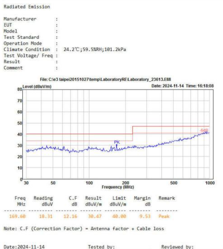
图 6-7 辐射测试垂直方向
