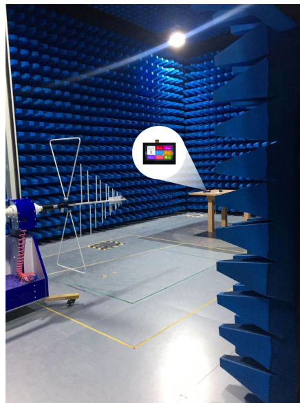
图 6-5 辐射测试图
